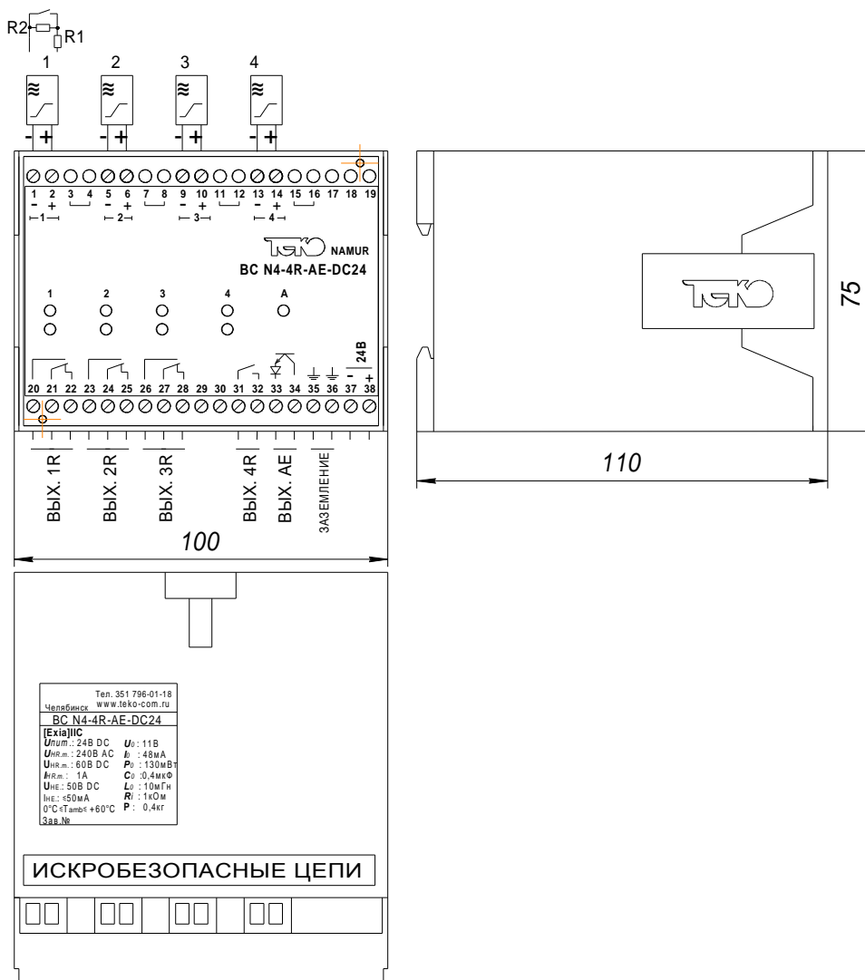
ГАБАРИТНЫЙ ЧЕРТЕЖ СХЕМА ПОДКЛЮЧЕНИЯ БЛОКА СОПРЯЖЕНИЯ
